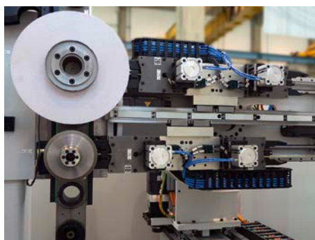
Automatischer Werkzeugwechsler
