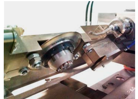
Schwenkabrichter
